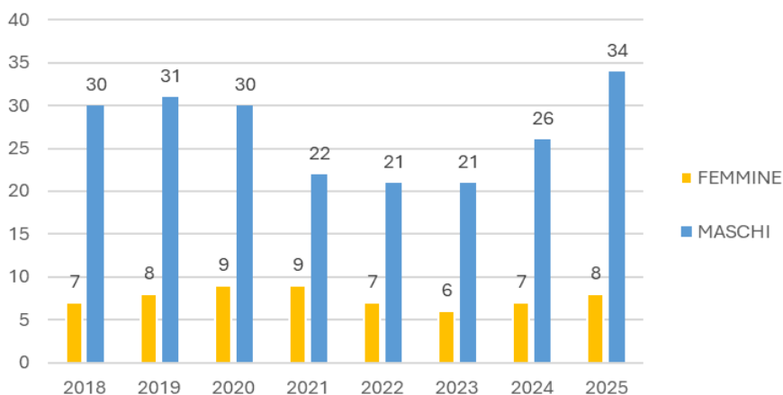
Composizione dipendenti
